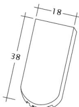
Технічне креслення черепиці SAKRAL FALZ
