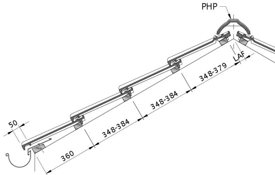
Технічне креслення черепиці CANTUS DQF DQF
