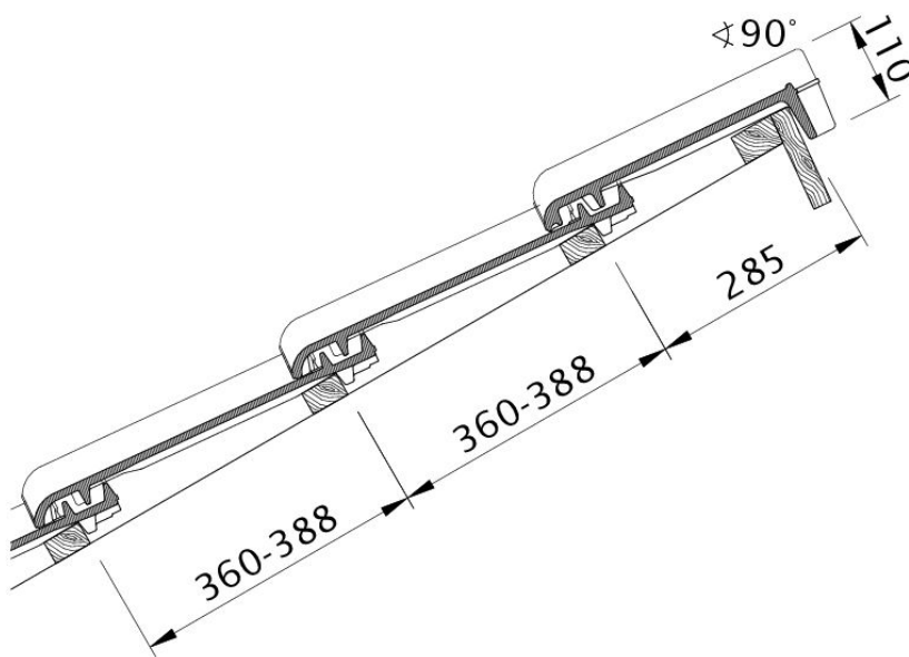
Технічне креслення черепиці FUTURA PDA PDA
