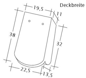
Технічне креслення черепиці KLASSIK LUEFTZ
