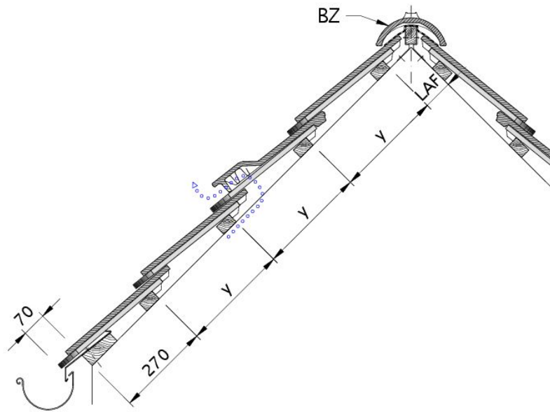
Технічне креслення черепиці KLASSIK DQF DQK-1
