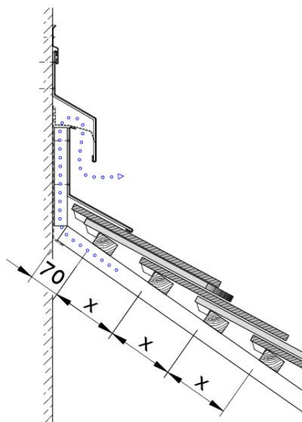
Технічне креслення черепиці KLASSEK WMF WMF-1
