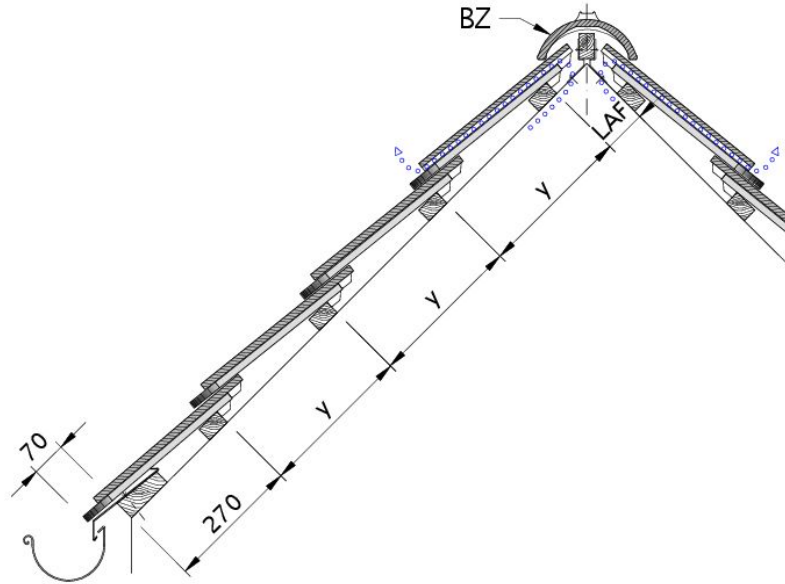
Технічне креслення черепиці KLASSIK DQF DQK-2
