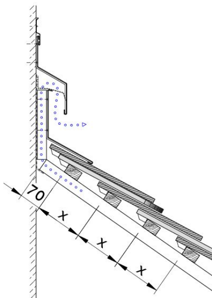
Технічне креслення черепиці KLASSIK WMF WMF-1
