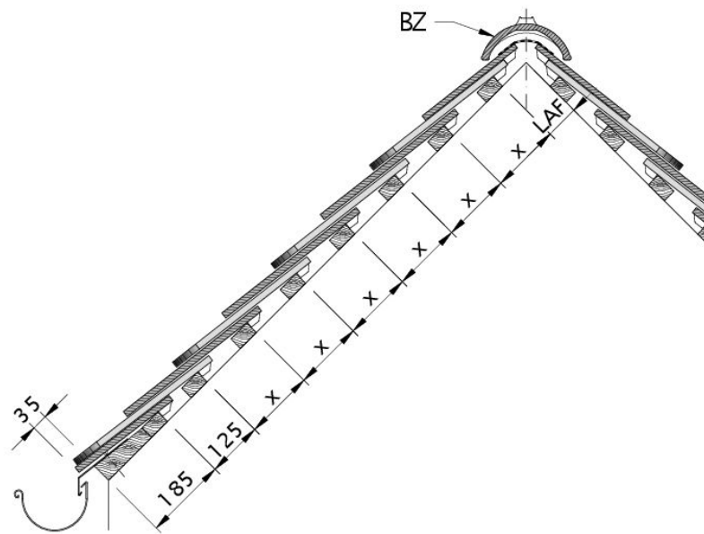
Технічне креслення черепиці KLASSIK DQF DQD-2
