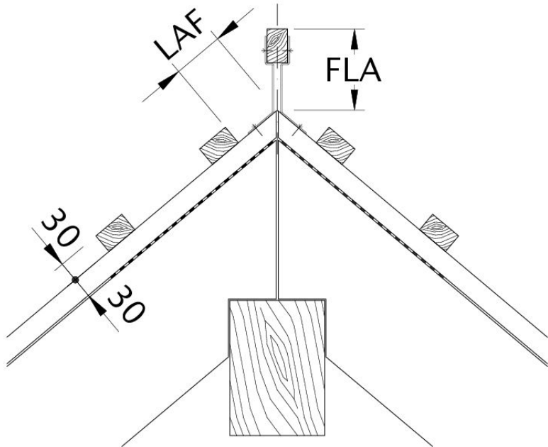
Технічне креслення черепиці KLASIK LAF LAF
